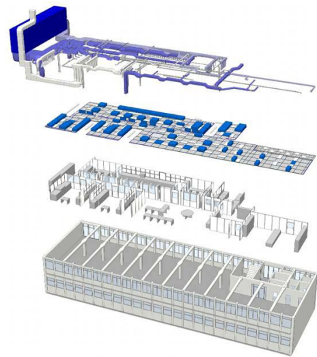
Beispiel eines Reinraumsystems von ASYS Cleanroom.
